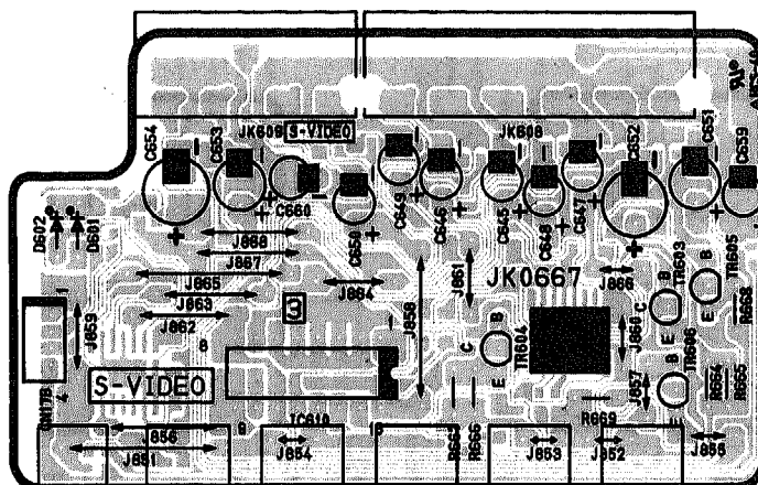
S-Video PWB
