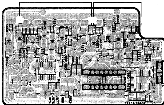
S-Video PWB
