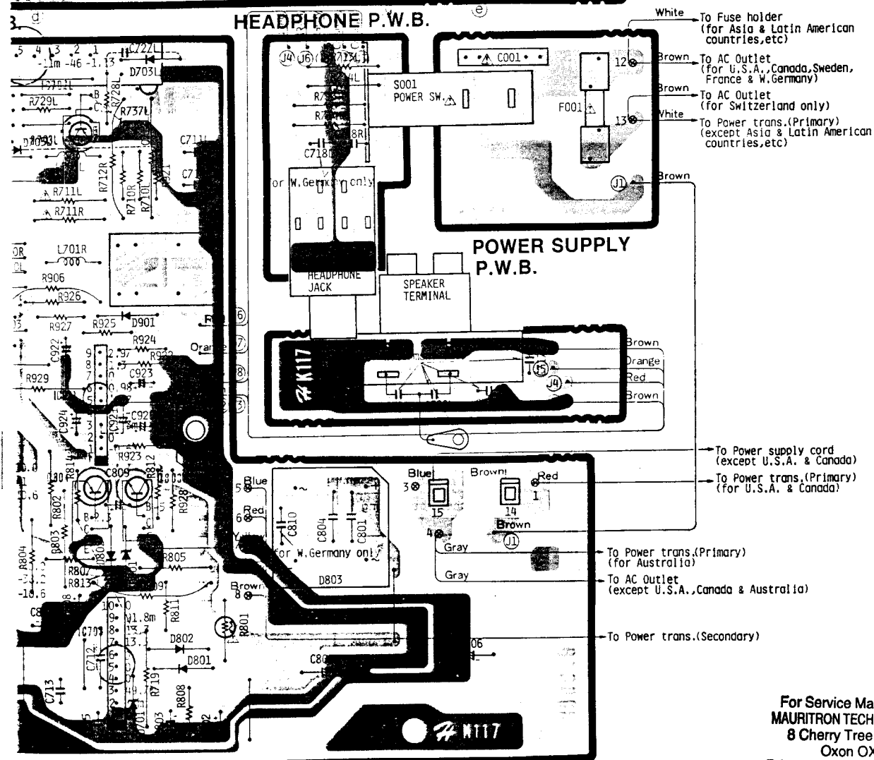
MAIN P.W.B.
