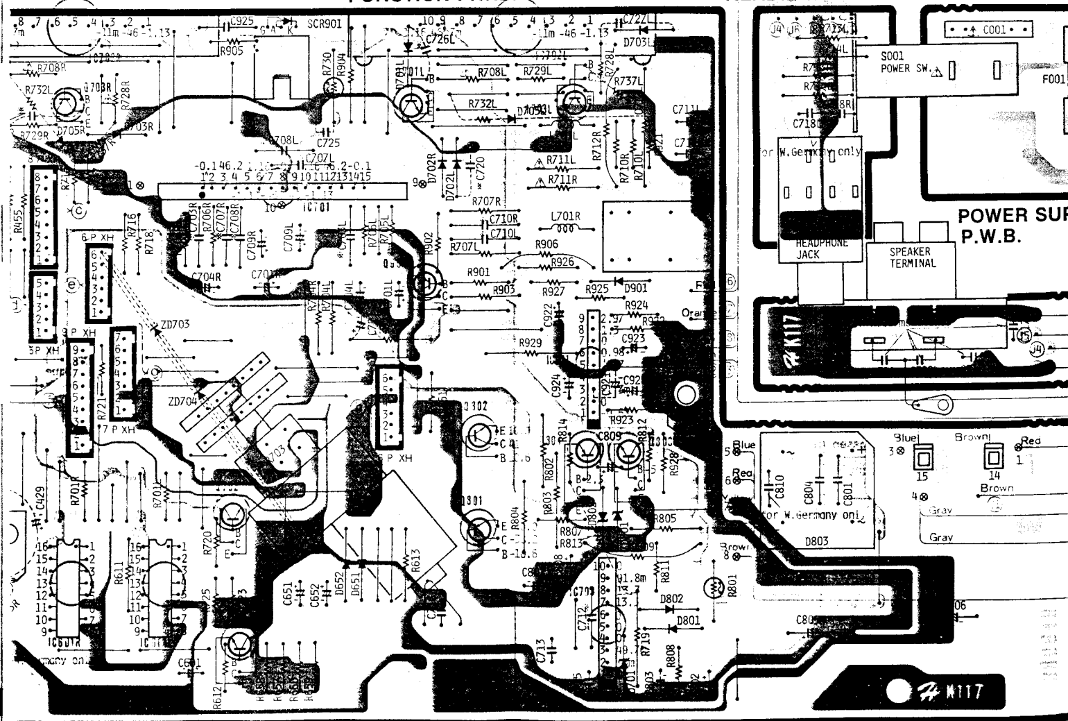
MAIN P.W.B.
