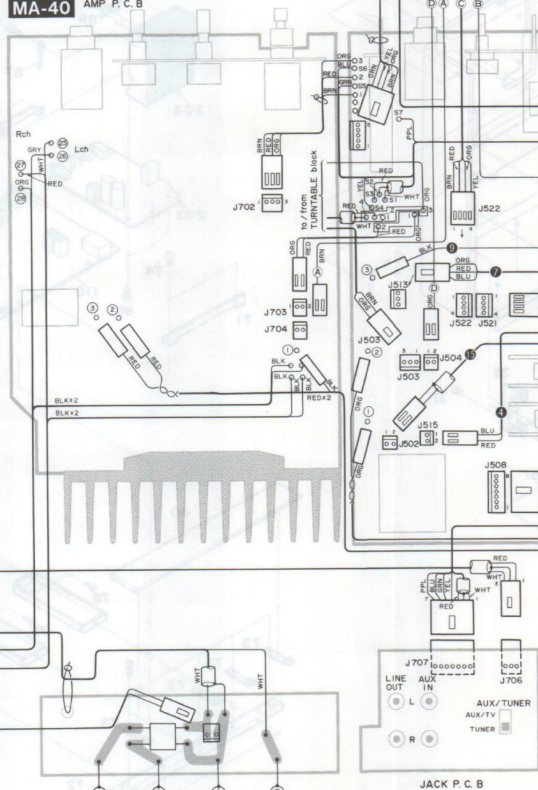
MA-40 AMP P.C.B
