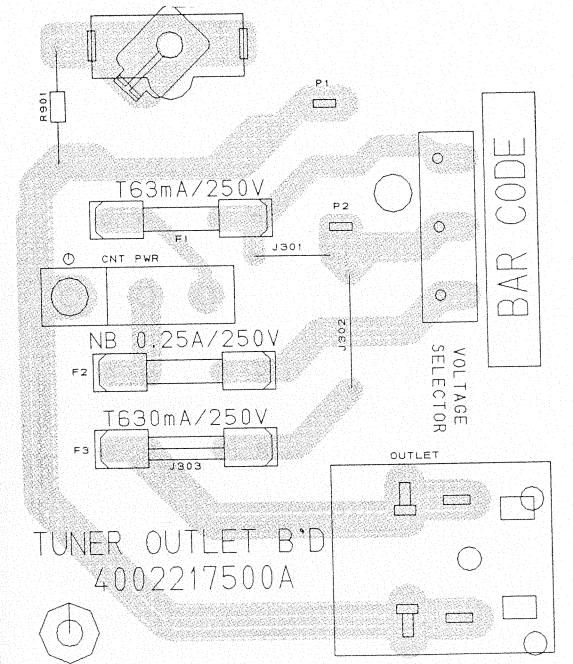
P.C.Board Tuner Outlet
