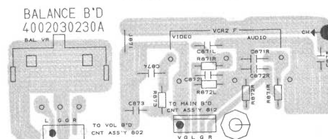
P.C.Board Balance
