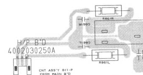
P.C.Board H/P
