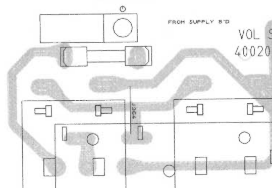
P.C.Board Vol. Sel.
