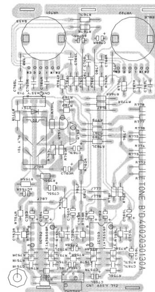
P.C.Board Tone
