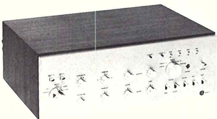
AMPLI E 200 2 x 35 W Distorsion par harmoniques inférieur à 0,2 %
