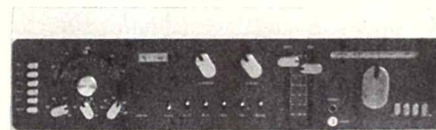
AMPLI TUNER PAT 30 2 x 22W sensibilité FM : 1 \mu V
