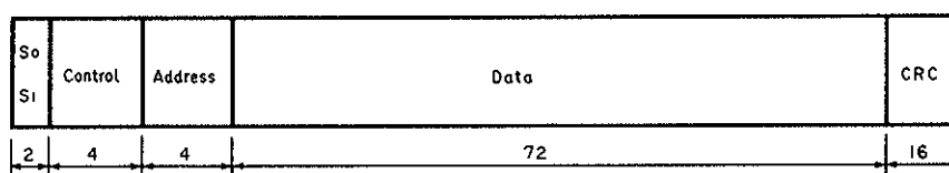
Fig. 45 Subcoding Q Format
