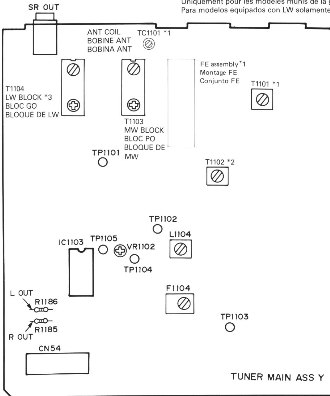
Fig. 6-2 Adjustment points Fig. 6-2 Points de réglage Fig. 6-2 Puntos de ajuste
