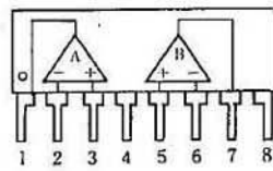
NJM4560L
