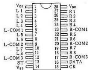
NJU7313AL
