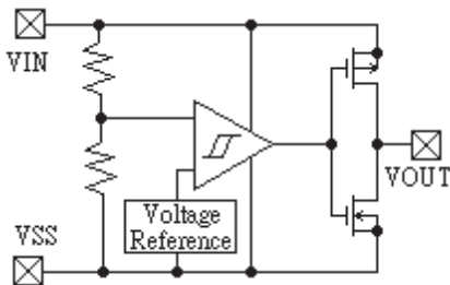
(1) CMOS Output
