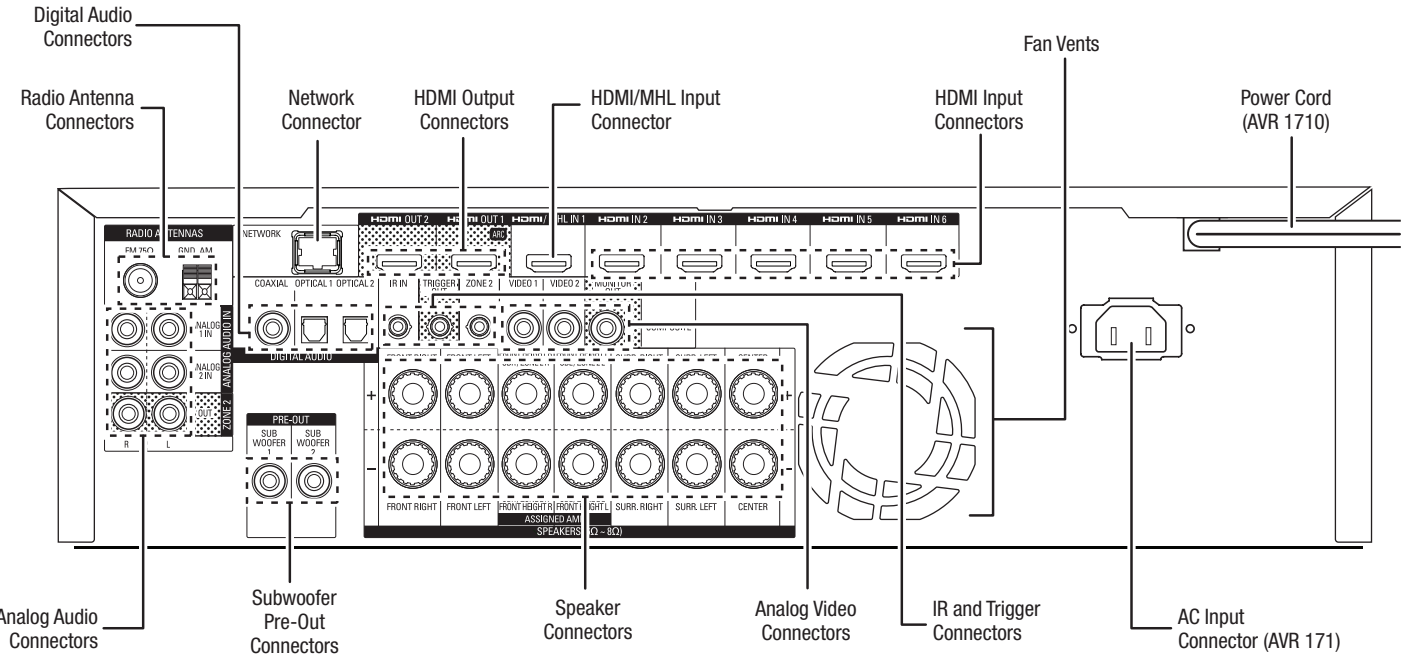
AVR 1710/AVR 171
