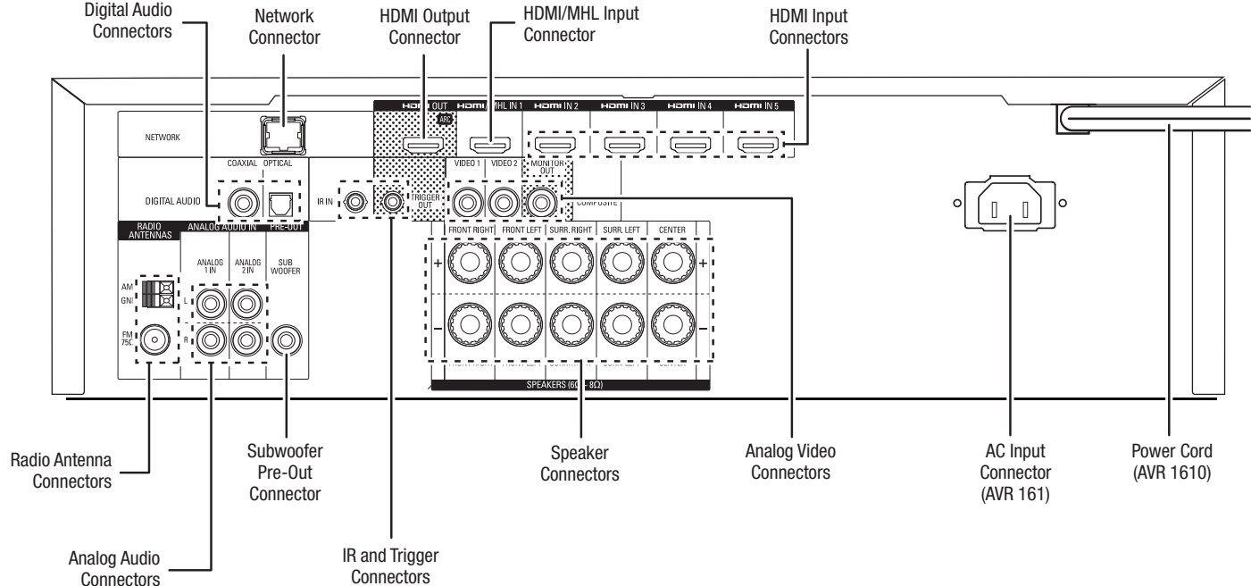
AVR 1610/AVR 161
