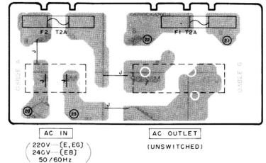
J AC IN/AC OUTLET P.C.B.
