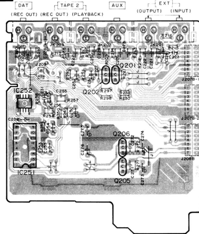
C INPUT/OUTPUT TERMINAL P.C.B.
