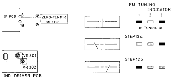
Fig. 4. FM Tuning Indicator Adjustment Abb. 4. UKW Abstimmmanzeige-Abgleich Fig. 4. Réglage de l'indicateur d'accord FM
