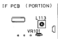
Fig. 3. FM Distortion Adjustment FM Signal Ind Calibration Abb. 3. UKW Verzerrung-Abgleich UKW Signalanzeige Eichung Fig. 3. Réglage de distorsion FM étalonnage de l'indicateur de signal FM
