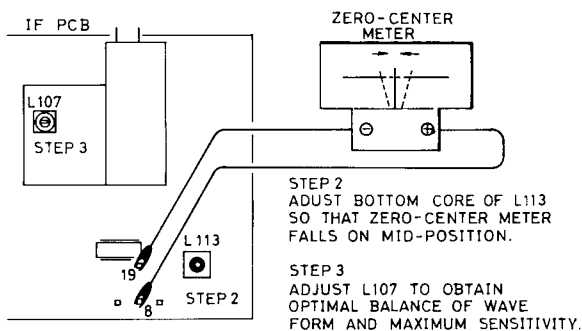
Fig. 1. FM IF Alignment Abb. 1. UKW-ZF-Einstellung Fig. 1. Alignement FM IF
