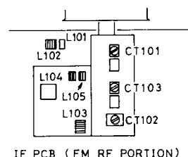
Fig. 2. FM RF Alignment Abb. 2. UKW-HF-Einstellung Fig. 2. Alignement FM HF
