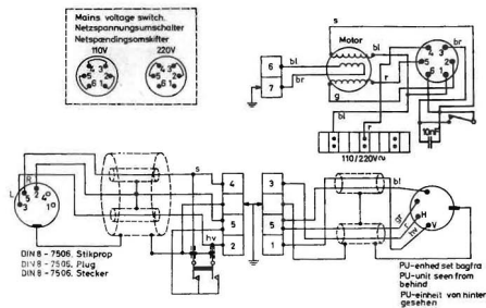
CIRCUIT DIAGRAM OF BEOGRAM 1200, TYPE 5214 / SCHALTBILD - BEOGRAM 1200, TYP 5214
