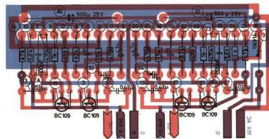
PC BOARD FOR TYPE 5306 / PRINTPLATTE FÜR TYP 5306
