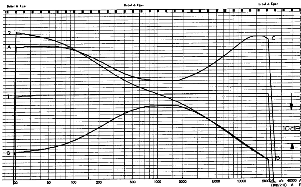
Frequenzgang 1 Eingänge RADIO, BAND 2 Phono-Entzerrung Wirkungsbereich der Klangregler A Bässe angehoben B Bässe abgesenkt C Höhen angehoben D Höhen abgesenkt
