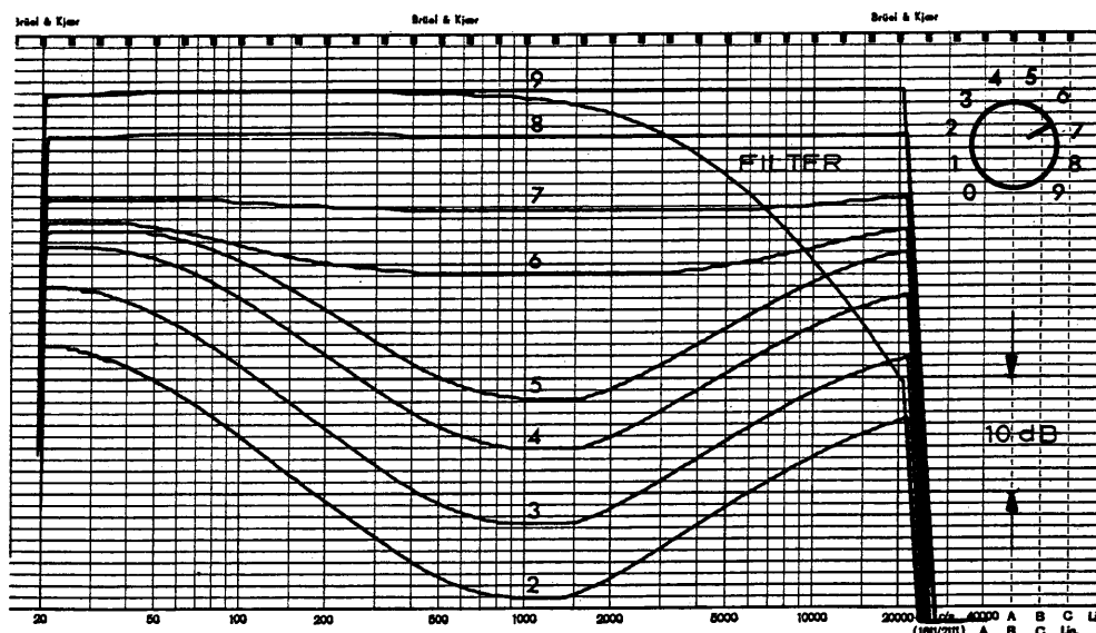
Frequenzgang Lautstärkeregl. (Contour) und Höhenfilter
