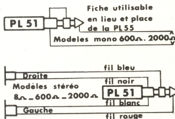
Schémas de branchement
