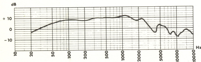
Courbe de réponse Amplitude/Fréquence
