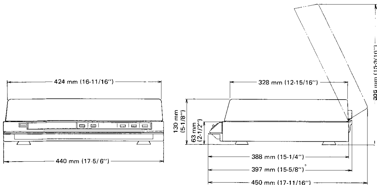
Fig. 1-1 Dimensions
