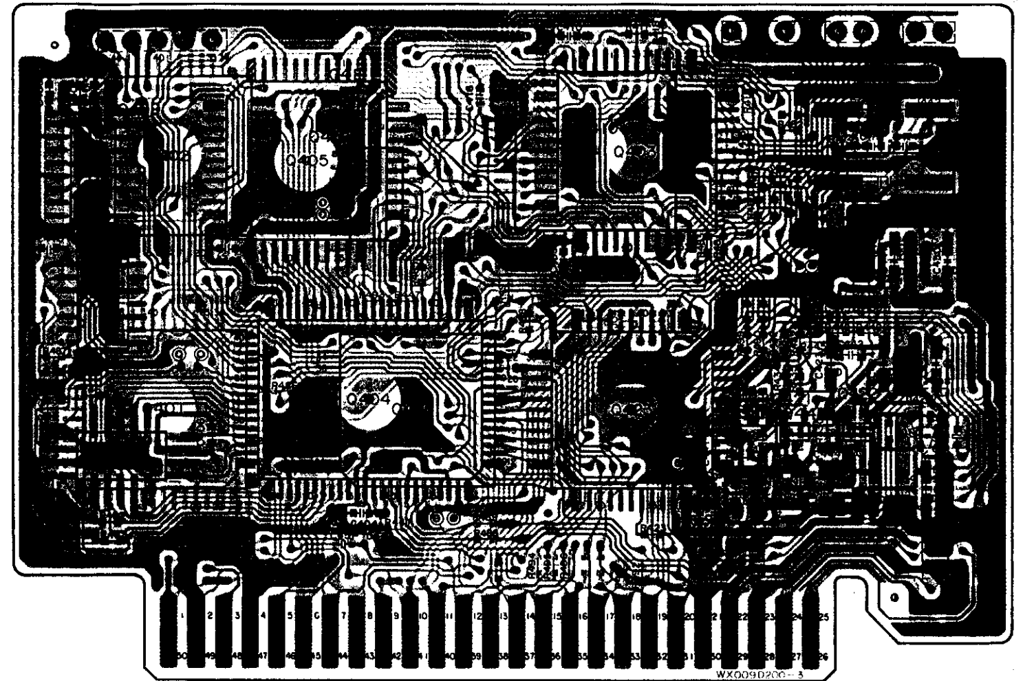
F PASC DIGITAL P.C.B. (ZZ01109010)
