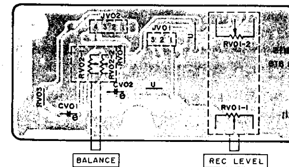
I REC LEVEL/ BALANCE P.C.B. (ZZ01102320)
