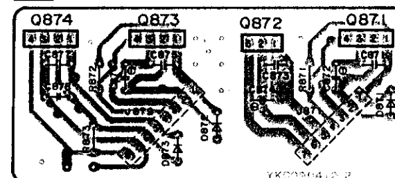
L REGULATOR P.C.B. (ZZ01104120)
