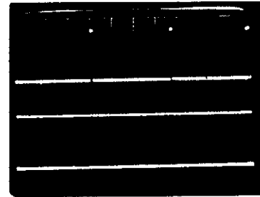
REC WITHOUT MUSIC SIGNAL Y : 0.2V × 10 X : 0.2ms
