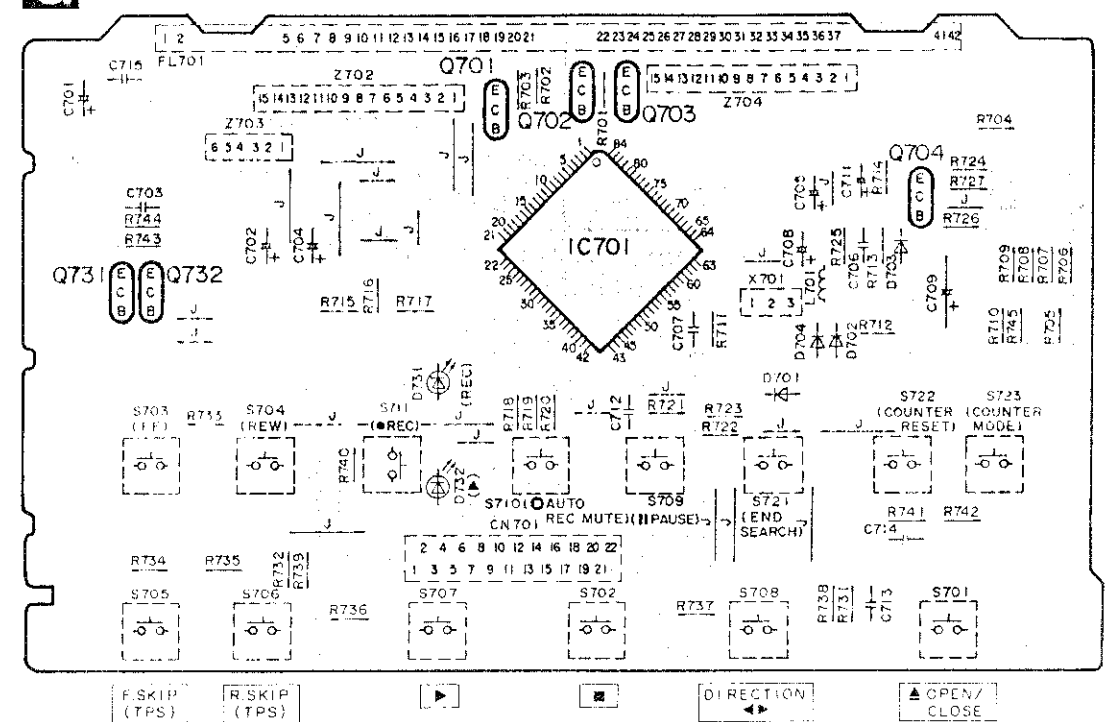
G FL P.C.B. (REPI702A-S)
