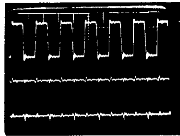
REC WITHOUT MUSIC SIGNAL Y : 0.2V × 10 X : 0.2μs
