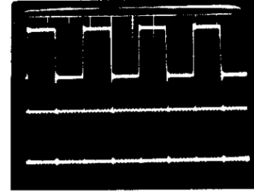
REC WITHOUT MUSIC SIGNAL Y : 0.2V × 10 X : 0.5μs
