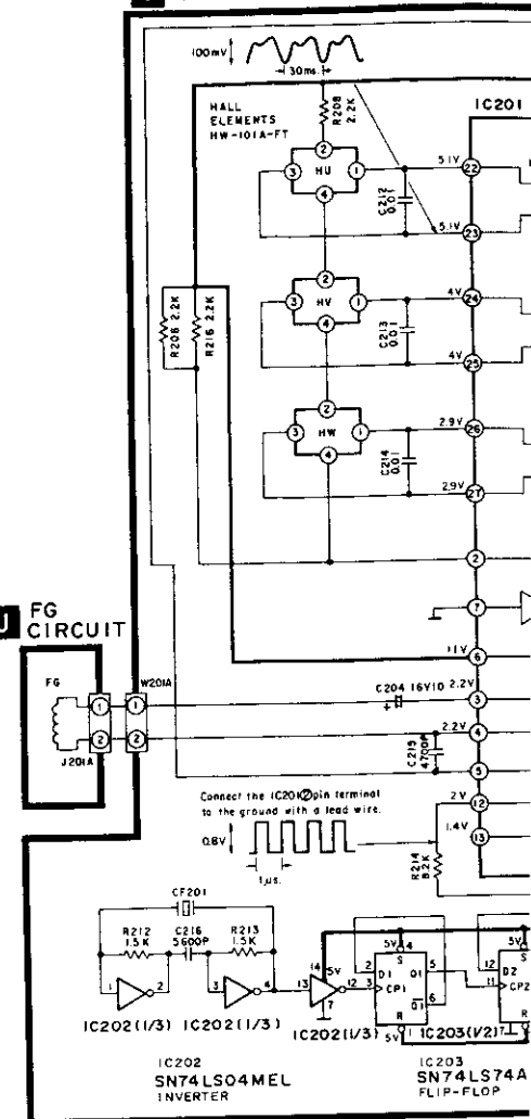
I CAPSTAN MOTOR(D.D.) CIRCUIT
