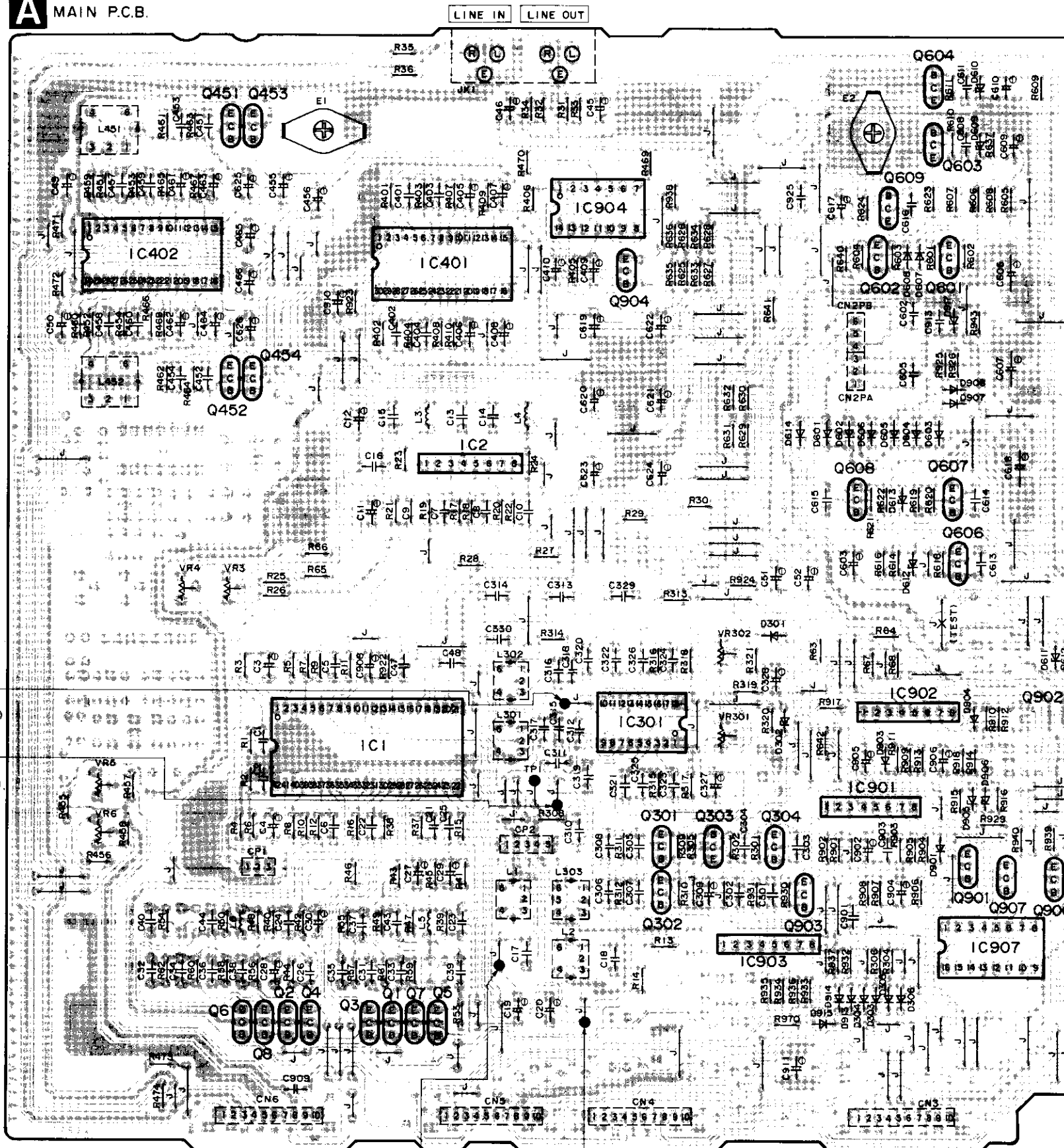
A MAIN P.C.B.
