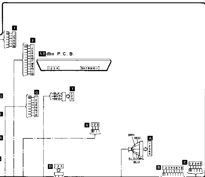
MAIN P.C.B.
