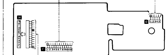
VOLUME/METER P.C.B.
