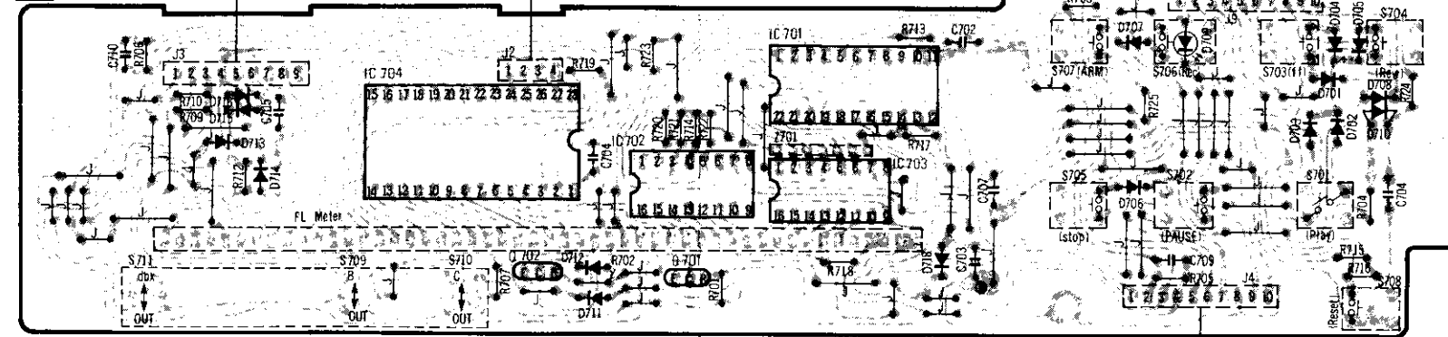
IV FL METER P.C.B.
