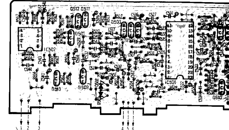
dbx P.C.B.
