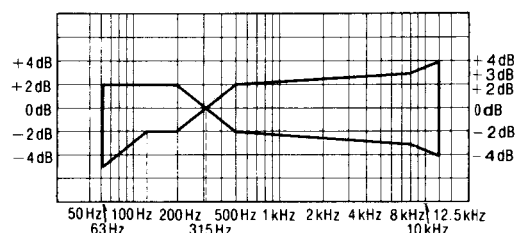
Wiedergabe-Frequenzgangsdiagramm
