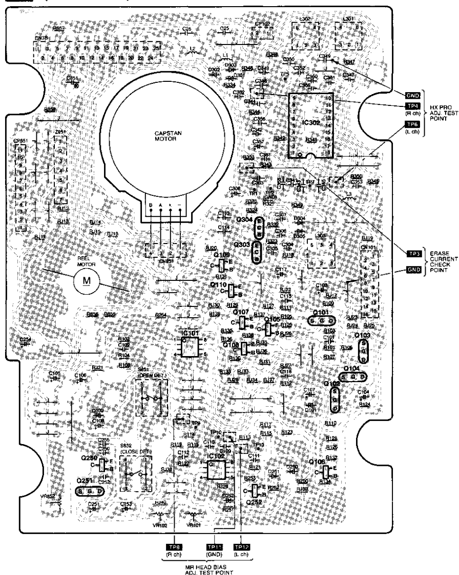
C MOTOR P.C.B. (REP2286A-T)
