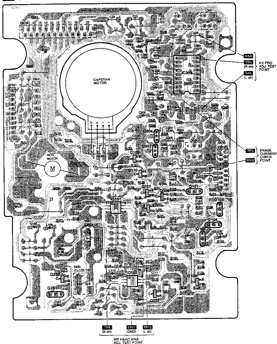
C MOTOR P.C.B. (REP2286A-T)
