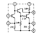
IC201 UPC1003C2
