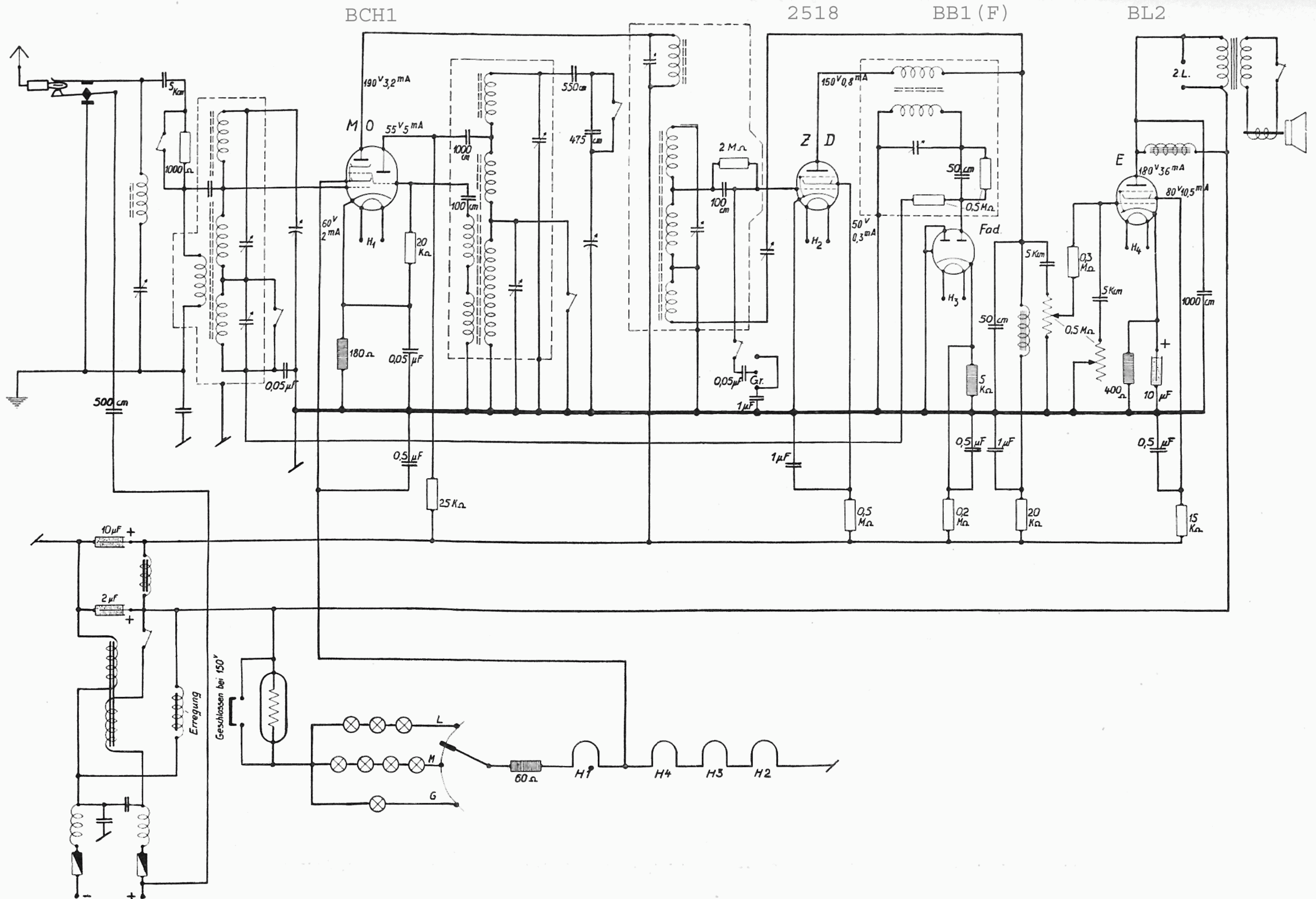
Dietz & Ritter, Miros GL, Gleichstrom, 1 Vorkreis, 2 Zwischenfrequenzkreise
