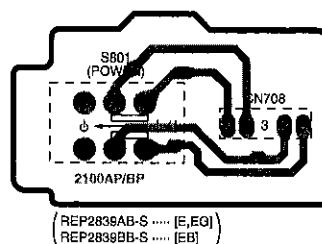
C POWER SWITCH P.C.B.
