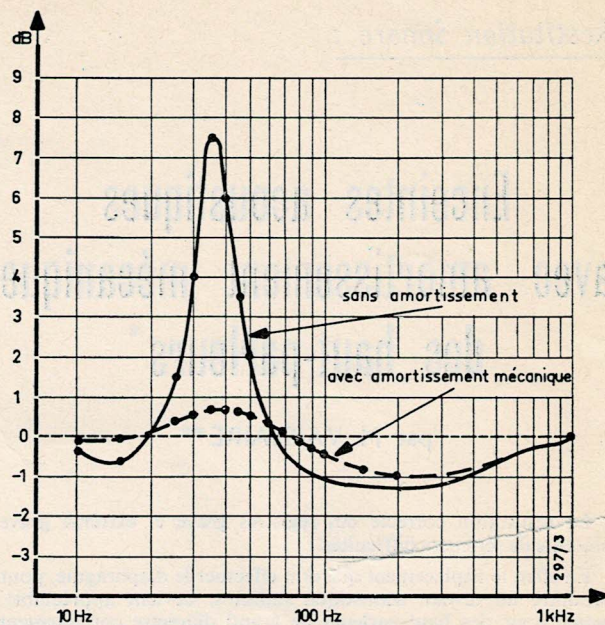
Fig. 3. — Tension aux bornes de la bobine mobile.
